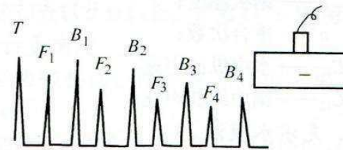
b) 缺陷F和底波B同时存在
