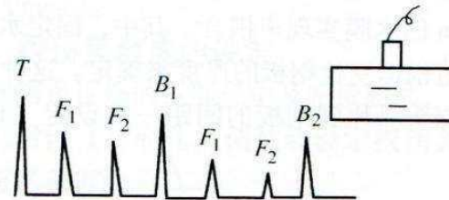
d) 一次底波内有二次缺陷波出现
