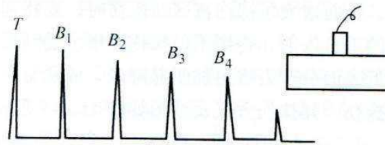
a) 钢板内只有底波B的多次反射，无缺陷
